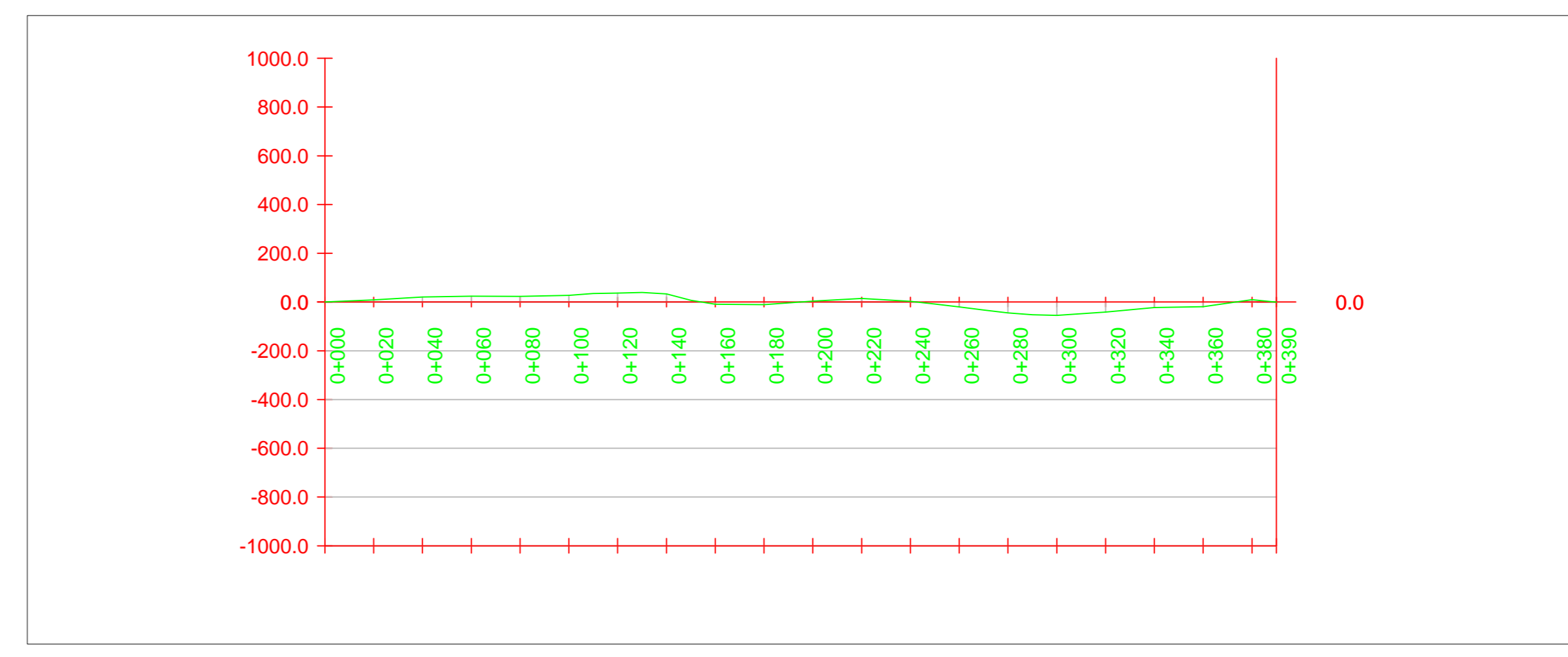
CURVA DE MASA TRAMO SECUNDARIO Abs. 0+000 - 0+390 Escala H---1: 2000 V---1:20000
